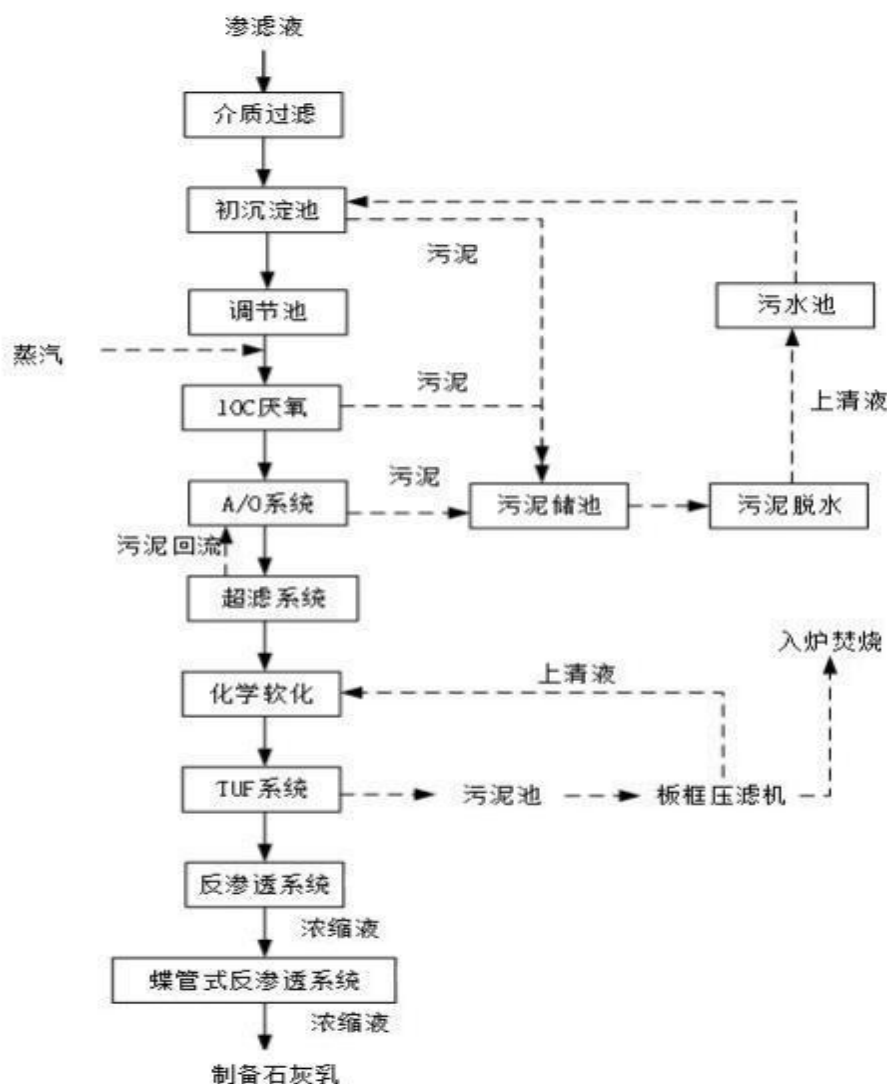
图 4-2 渗滤液处理站工艺流程图
