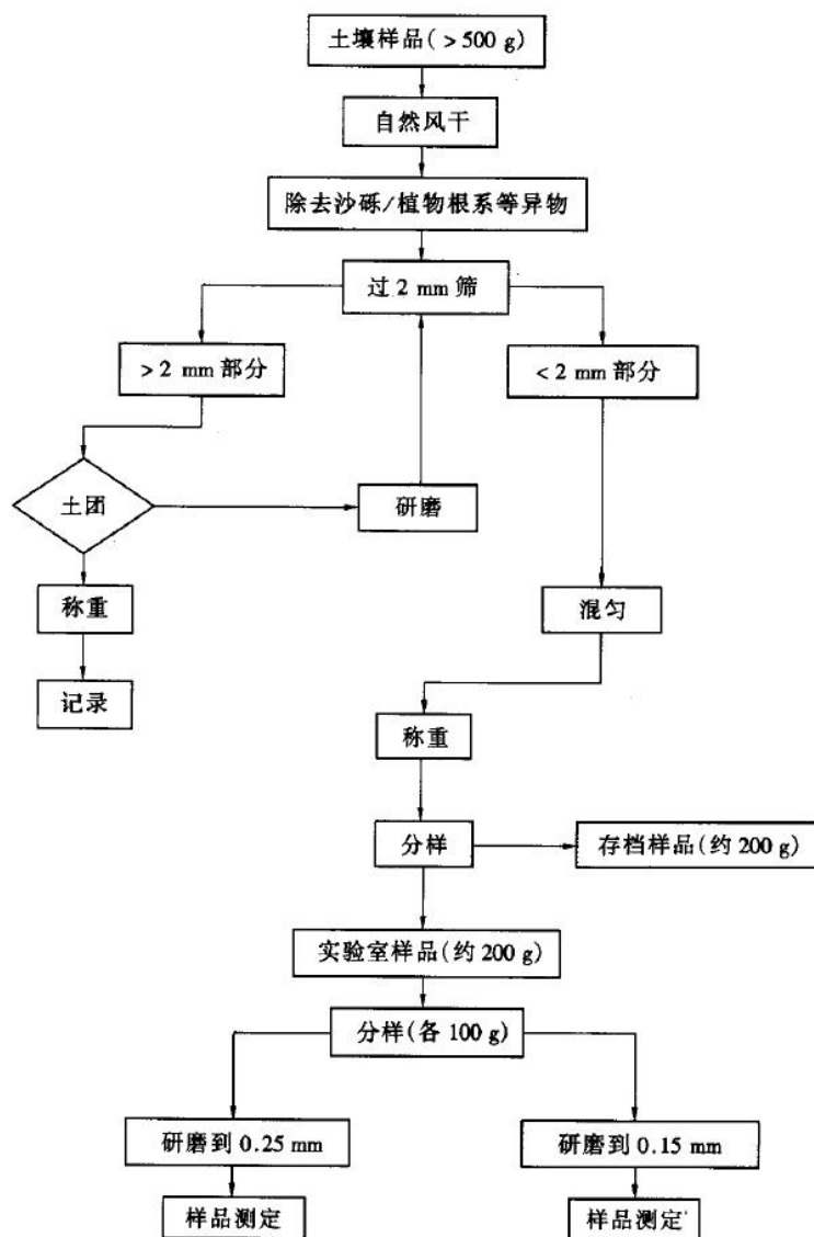
图 7-1 土壤制样过程
