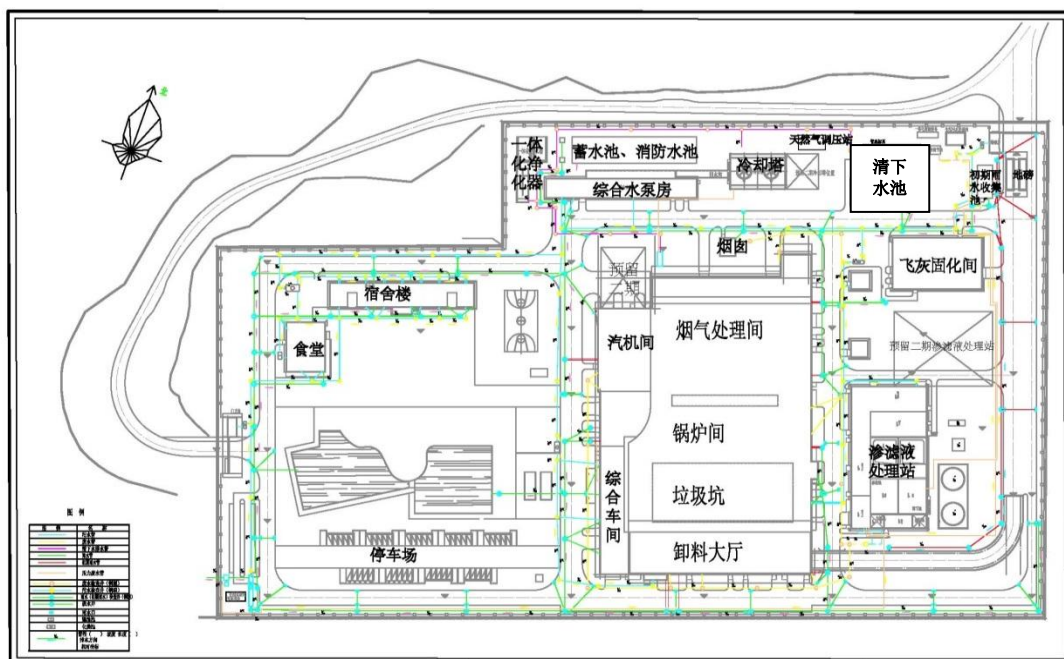
图 4-3 厂区平面布置图
