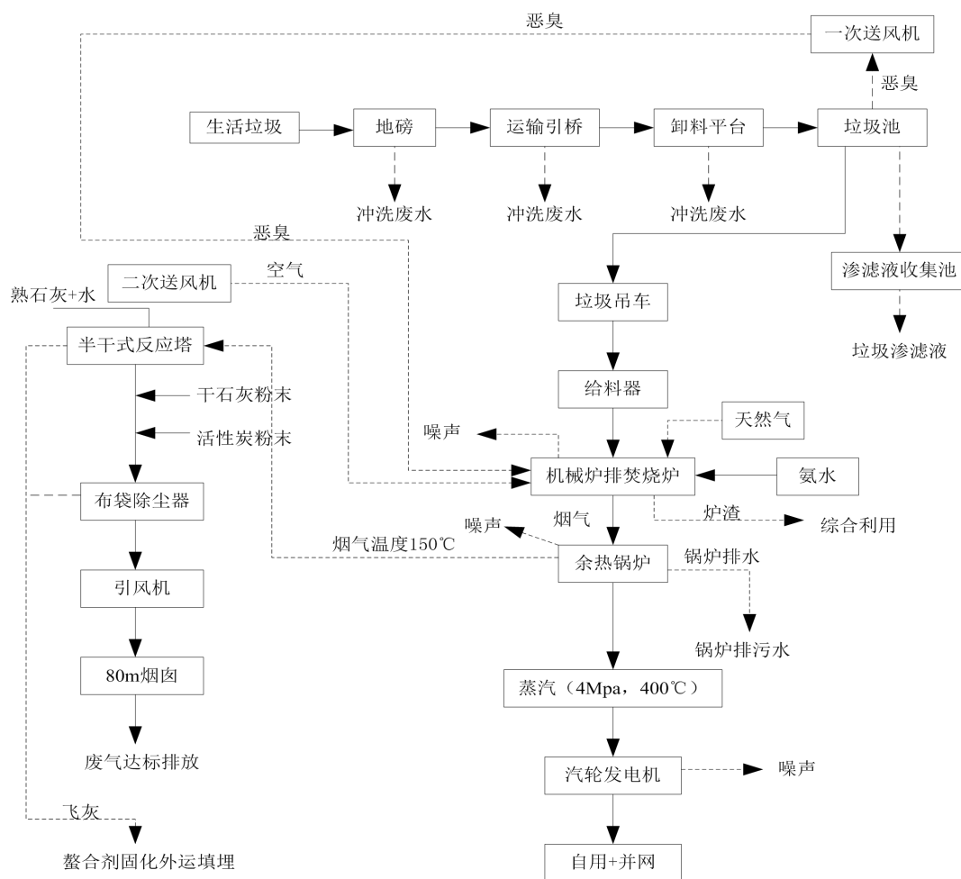
图 4-1 生产工艺流程图
