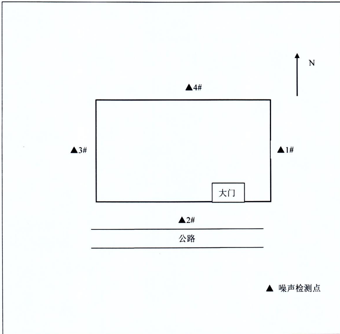
图 5-1 检测布点图
